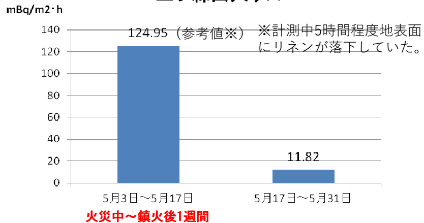
リネン吸着法 (Cs合計 \text{mBq}/\text{m}^2\cdot\text{h} ) 三ツ森山入り口
